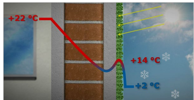
Gradient de température chimique avec ThermoProtect en hiver. Gain solaire de 12 °C.
